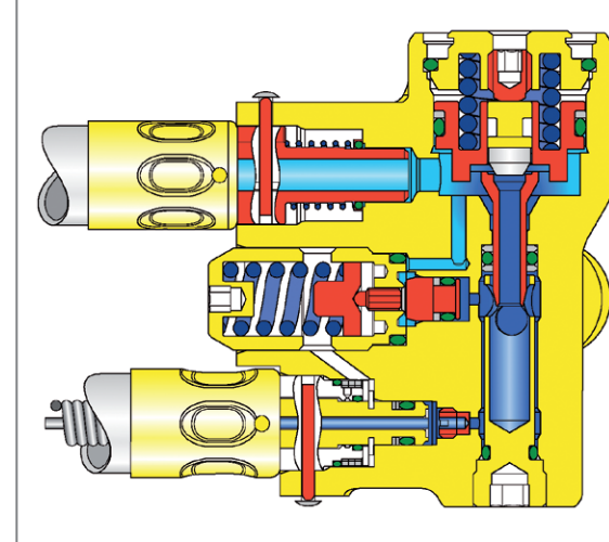
Manorreductor cargado, sin flujo de aire
