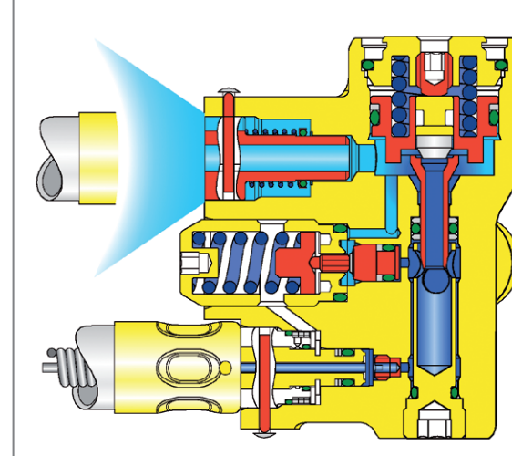
Válvula de seguridad abierta
