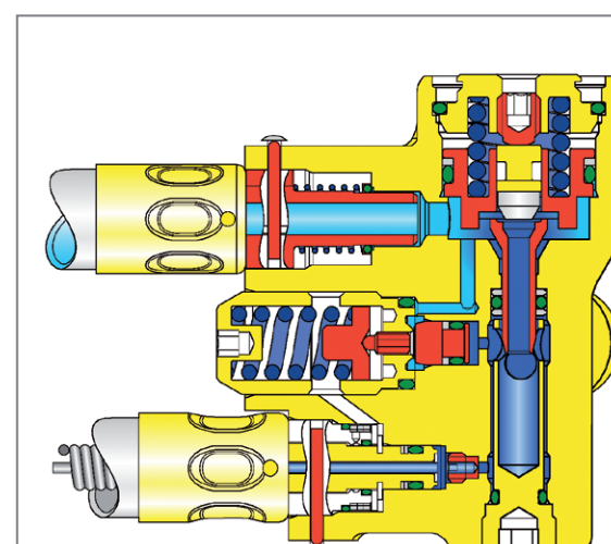
Manorreductor cargado, con flujo de aire
